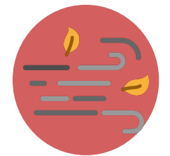
de wind
